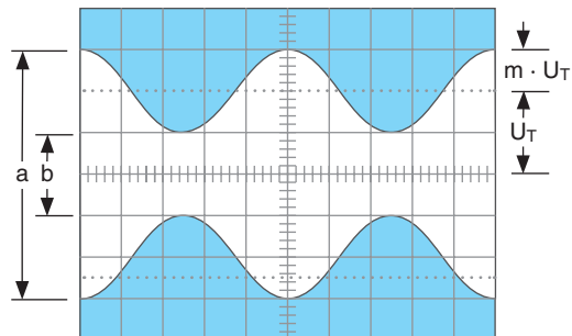
Abb. 2 Amplitudenmodulierte Schwingung: F = 1 MHz; f = 1 kHz; m = 50%; U_T = 28,3 \text{ mV}_{\text{eff}} .
